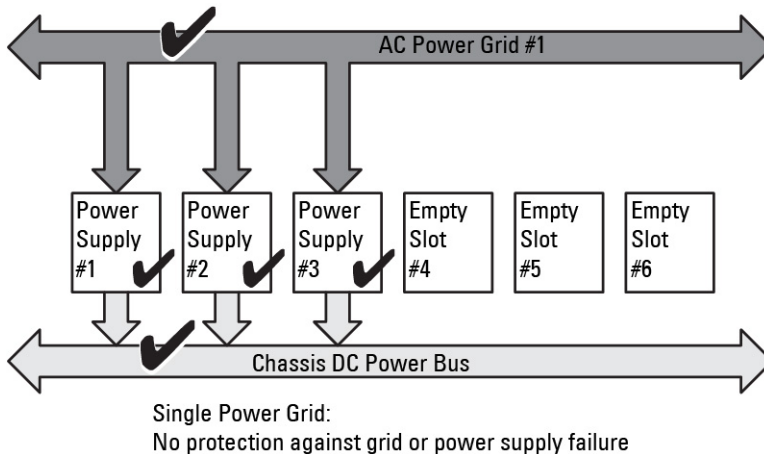
图 7: 机箱中 3 个 PSU 且无冗余
